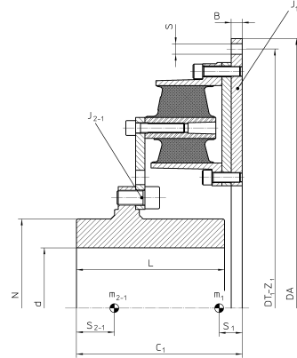
Series TFS1-Hub 3 - Bauform TFS1-Nabe 3
