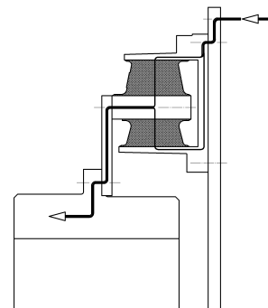
Flow of torque Drehmomentfluss
