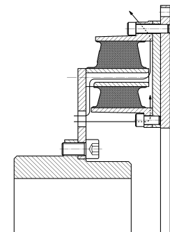
Internal air flow for good heat dissipation / Interner Luftstrom für gute Wärmeableitung
